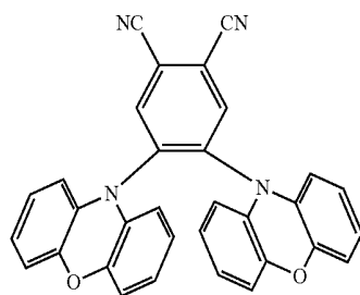
(PXZ) 2 PN
