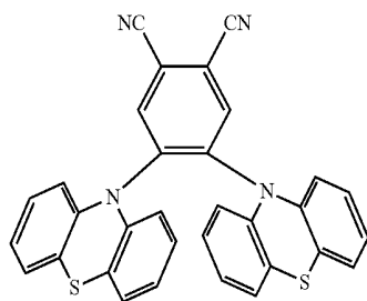
(PTZ) 2 PN
