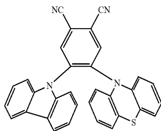
CzPTZPN
