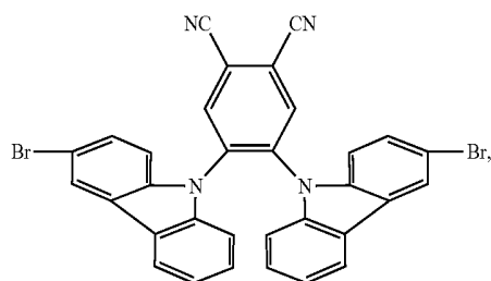
(3-BrCz) 2 PN
