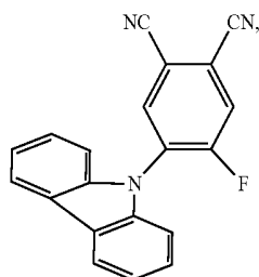
CzFPN
